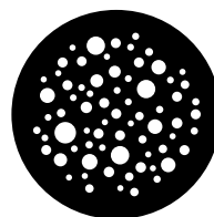
品号:190320000097 外径:Ø32.0 图案:Ø26 厚度:1.1mm 位置:6
